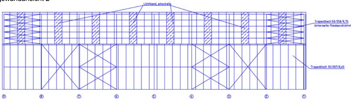
Längswandansicht 2
