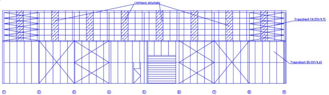
Längswandansicht 2
